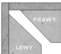
Narożnik zewnętrzny 90° dwuelementowy 100x112cm
